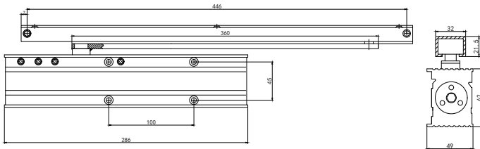
凸轮结构 Cam Action
